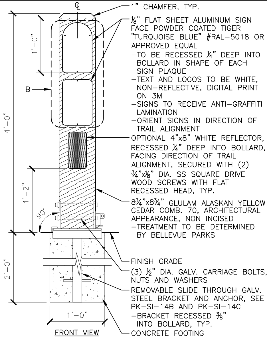
A-BOLLARD DETAIL
